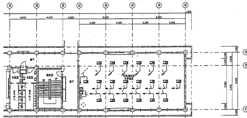
【第3教棟】4階平面図 1/150 【改修後】
