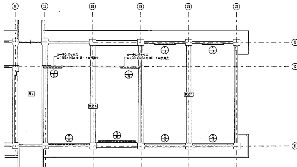
【第3教棟】4階 教室4・教室5 撤去カーテン位置図 1/100
