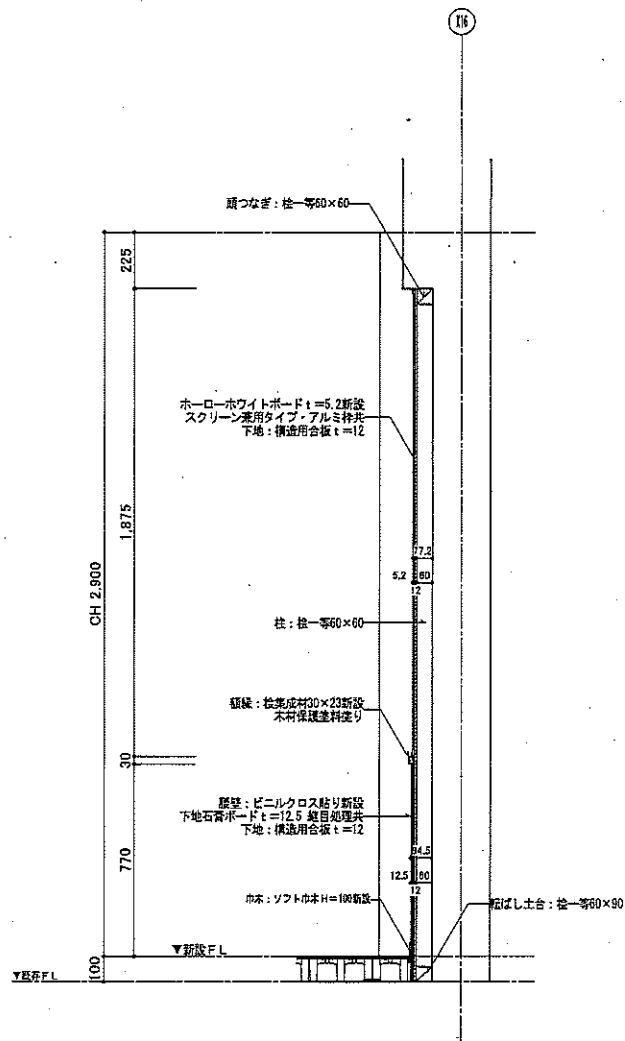
ホワイトボード詳細図 (2) 1/15
