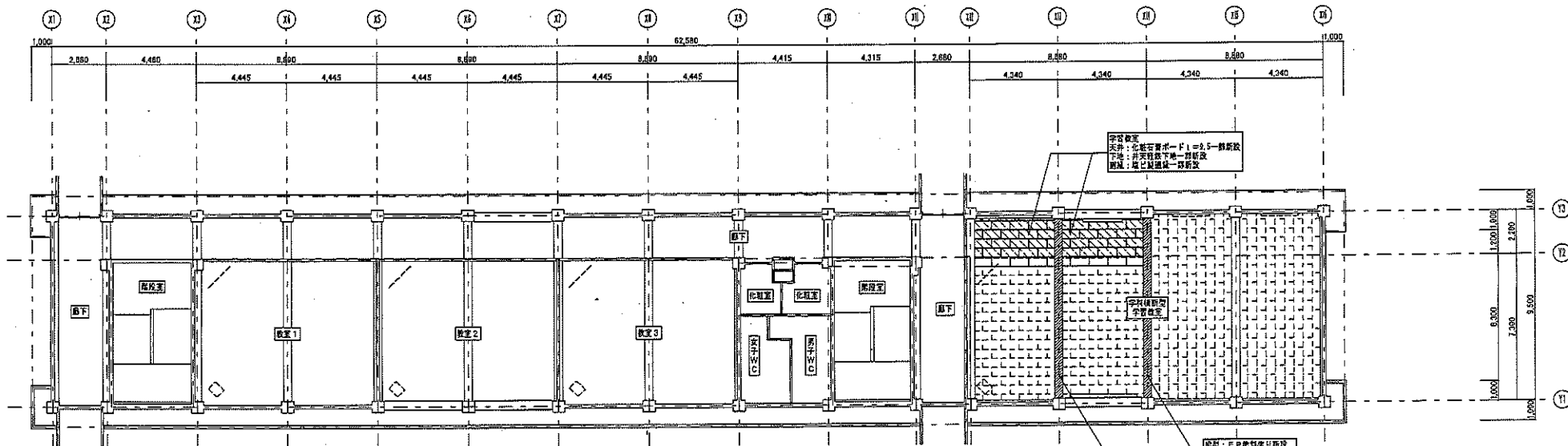
【第3教棟】4階天井伏図 1/150 〔改修後〕
