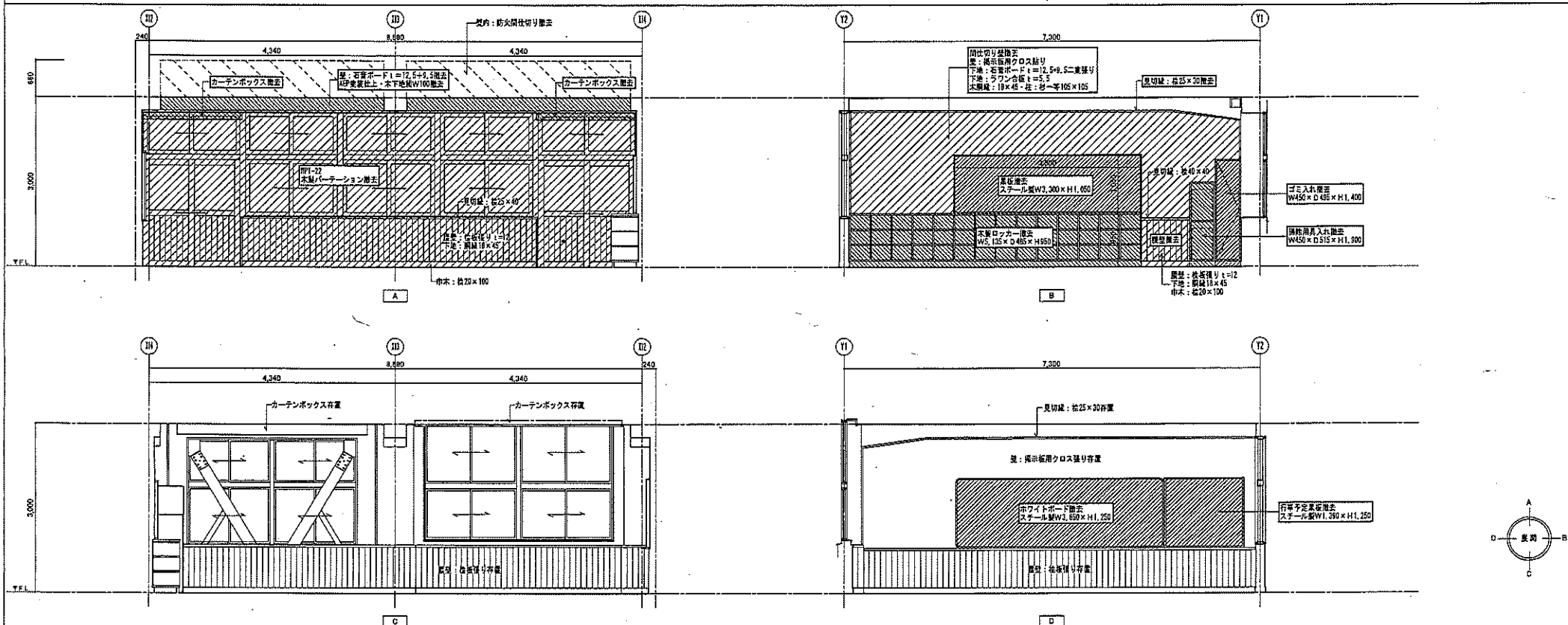
【撤去】第3教棟 4階 教室4 1/50
