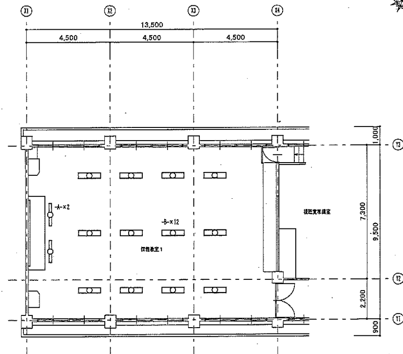
【第1教棟】3階平面図 1/100 [改修後]
