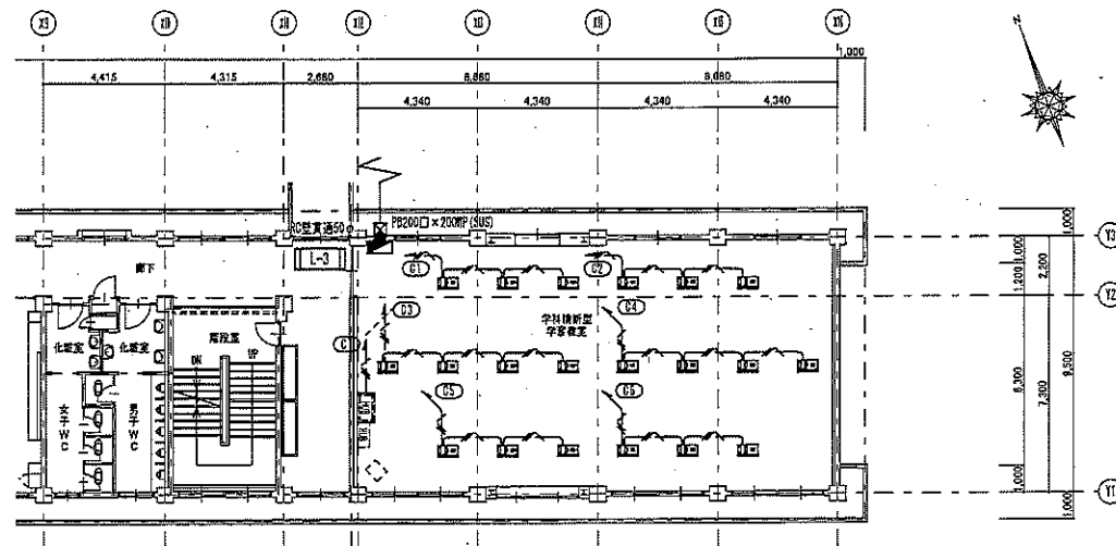
【第3教棟】4階平面図 1/150 【改修後】
