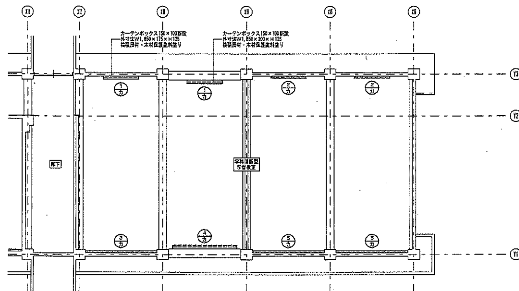
【第3教棟】4階 学科横断型学習教室 改修カーテン位置図 1/100
