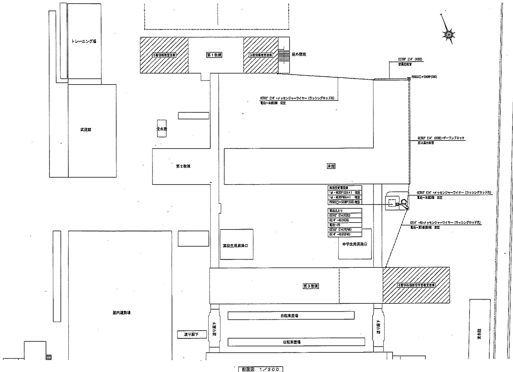
配置図 1/300
