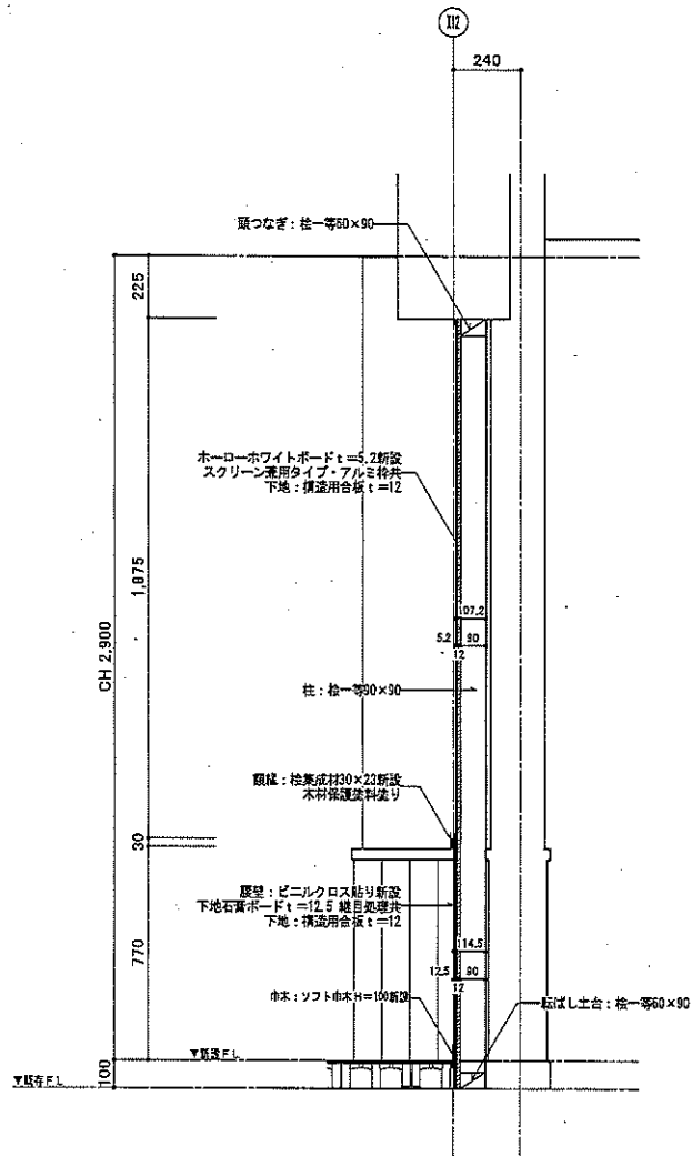
ホワイトボード詳細図 (1) 1/15
