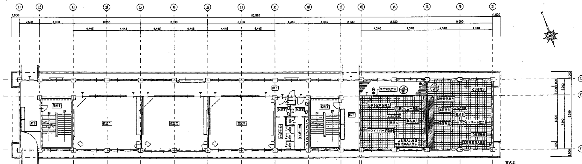
【第3教棟】4階平面図 1/150 【改修前】
