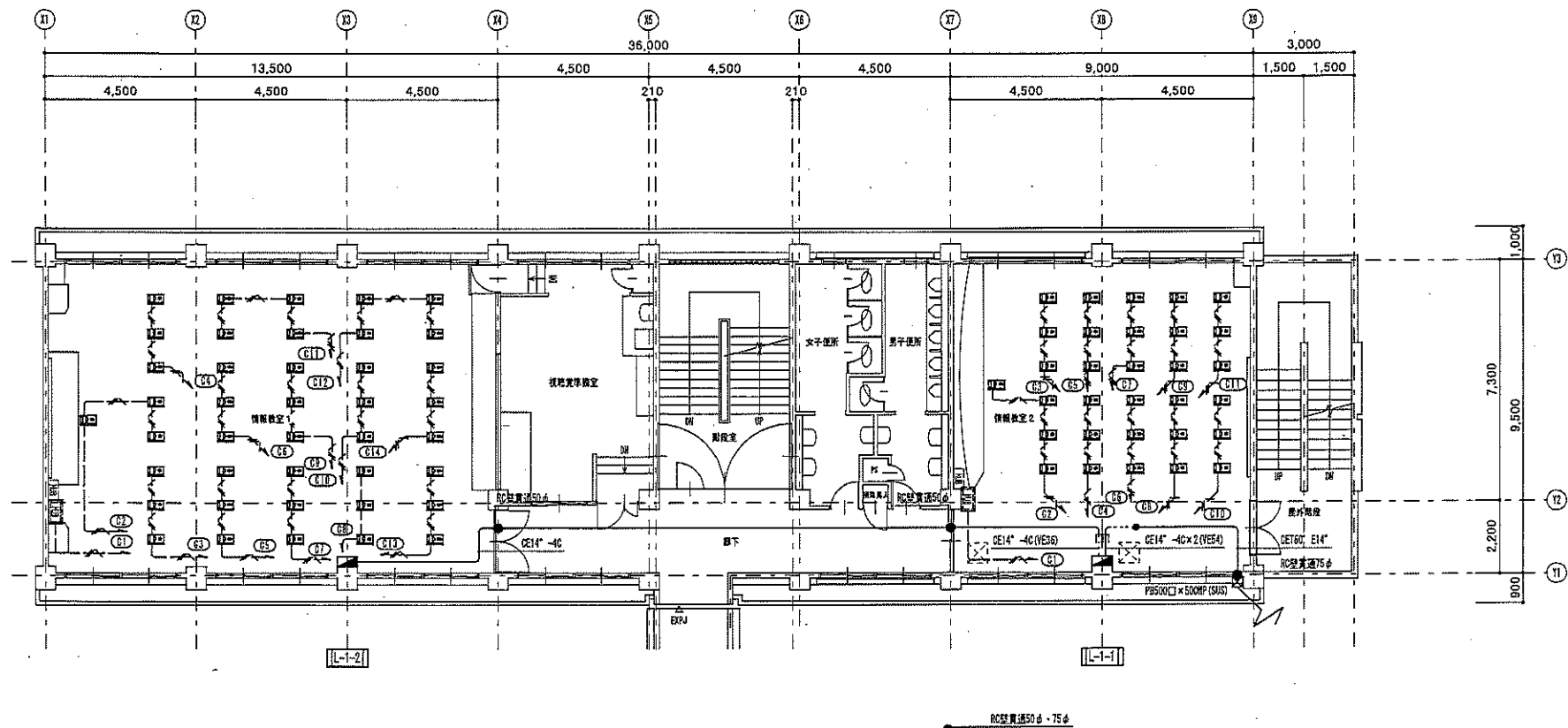
【第1教棟】3階平面図 1/100 【改修後】
