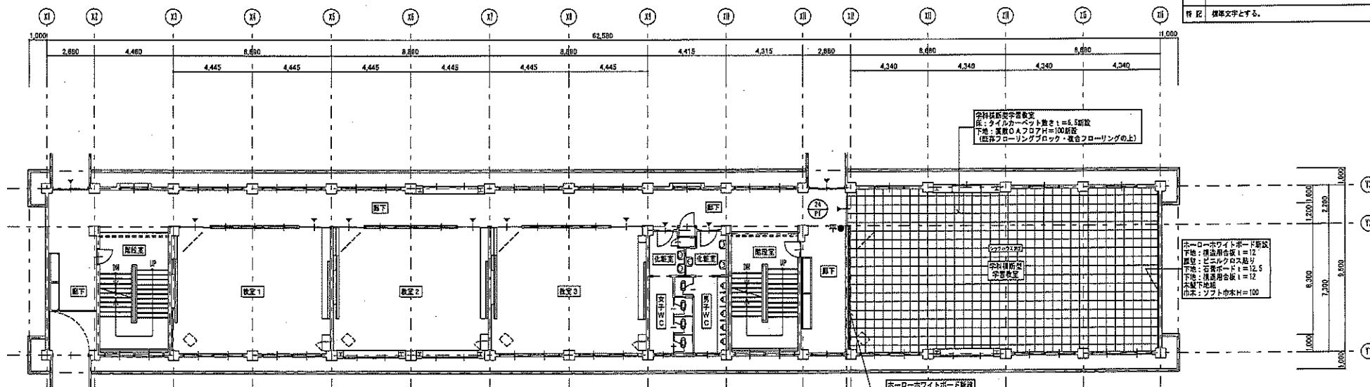
【第3教棟】4階平面図 1/150 【改修後】
