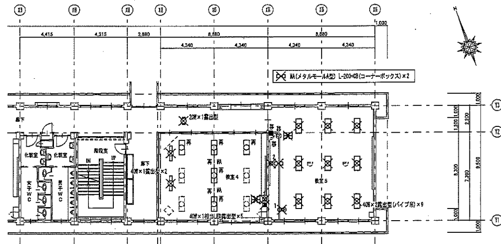
【第3教棟】4階平面図 1/150 【改修前】
